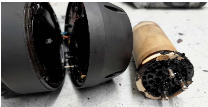
Poškodenie spôsobené vonkajšími výparmi
