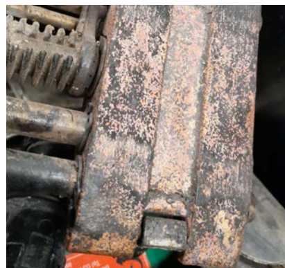
ホットウェッジ 頻繁な溶接による摩耗。溶接温度が最高値に設定されている。
