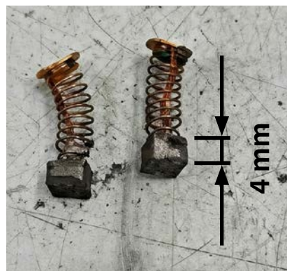
カーボンブラシ 通常使用による摩耗。残り長さが4 mmになるとカーボンブラシストップが作動します。
