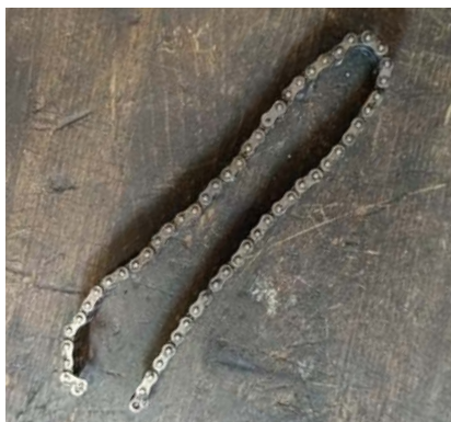
チェーン 過度の圧力による損傷。
