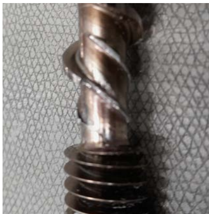
Uso improprio: Piccoli detriti, trascinati dal filo di saldatura, hanno danneggiato la vite.
